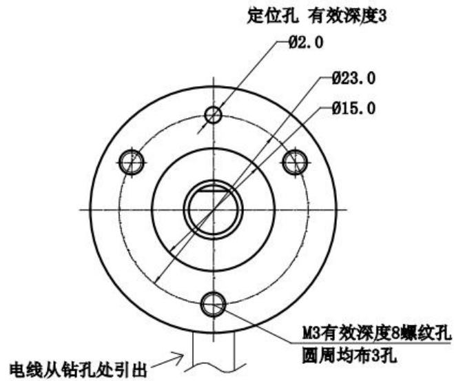
壳体安装面
