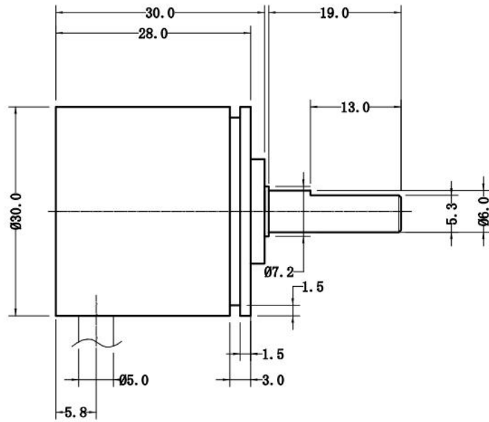
壳体侧面
