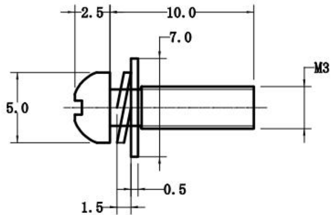
配件(组合螺丝 M3*10)
